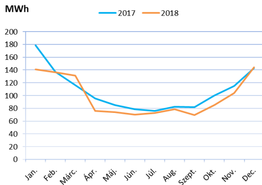
2. ábra Villamosenergia-felhasználás
