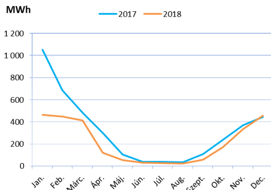
3. ábra Gázenergia-felhasználás
